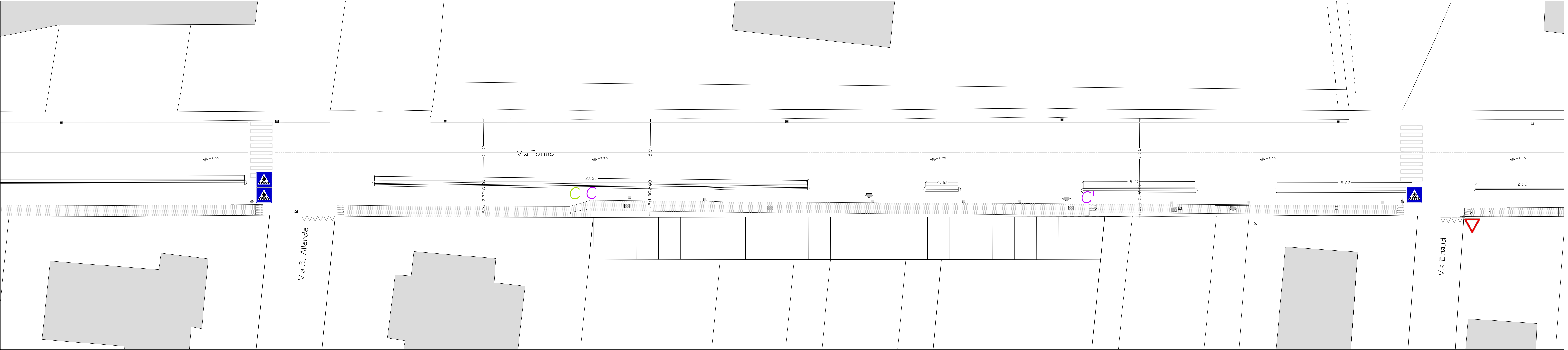
TRATTO AB QUADRO 2 -Scala 1/200
